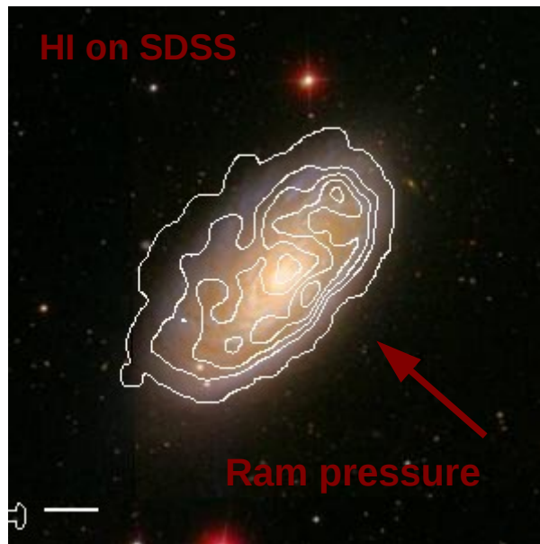
NGC 4501
